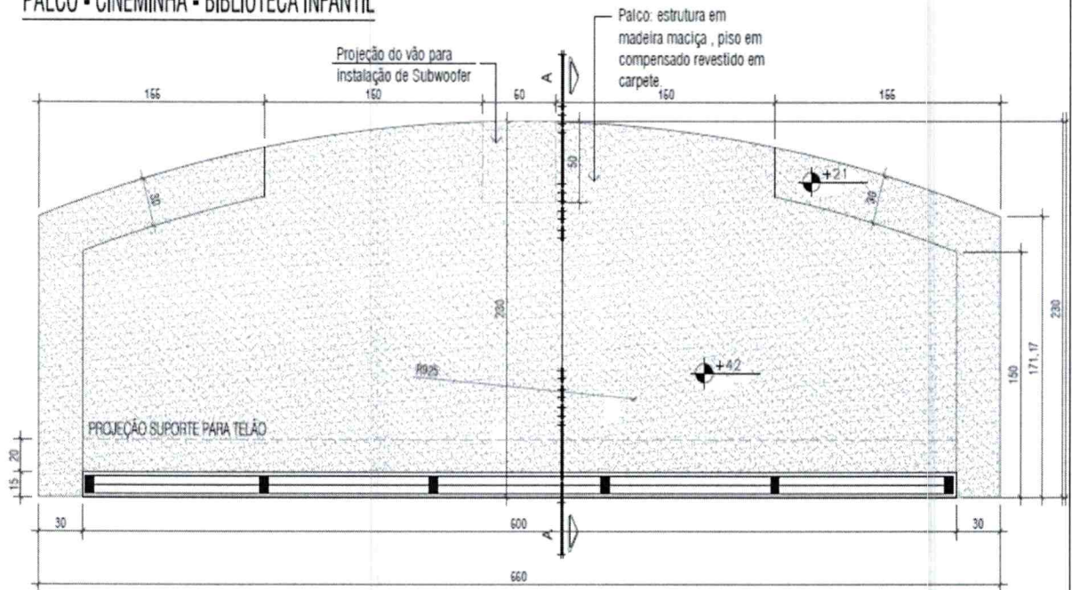
PLANTA BAIXA PALCO - BIBLIOTECA INFANTIL esc:1/25
